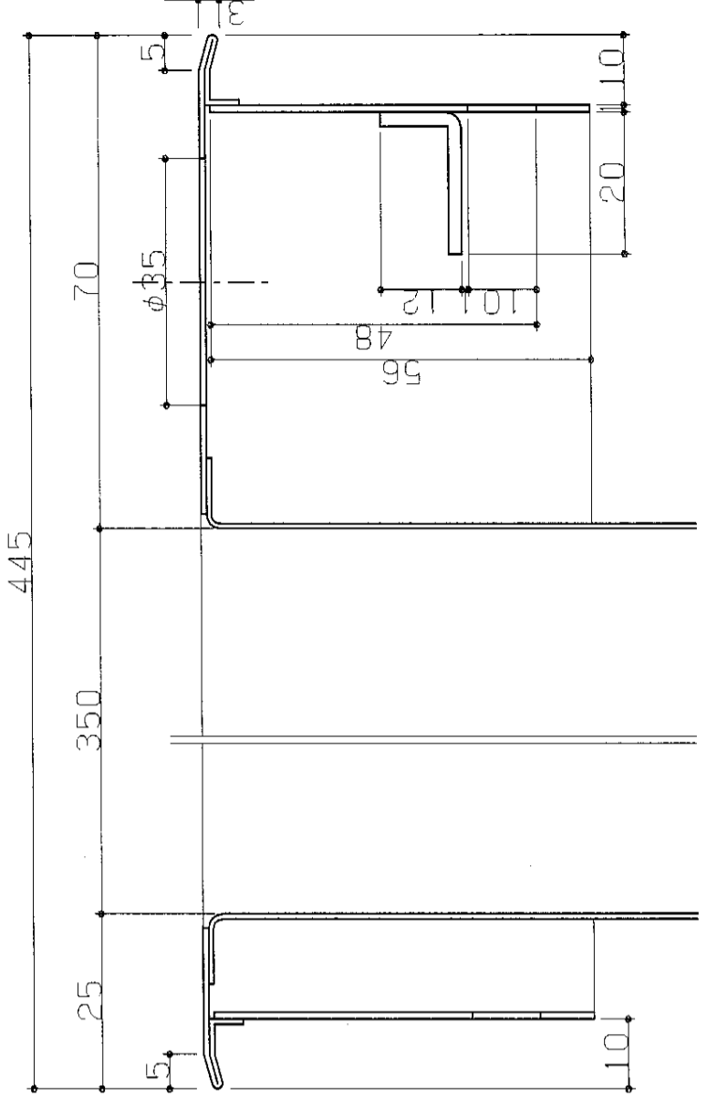
BB断面(1/1)
