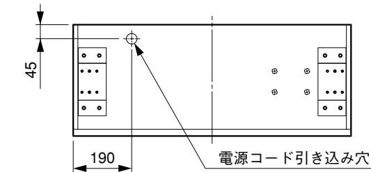
上面図
