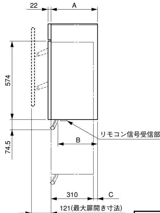
側面図
