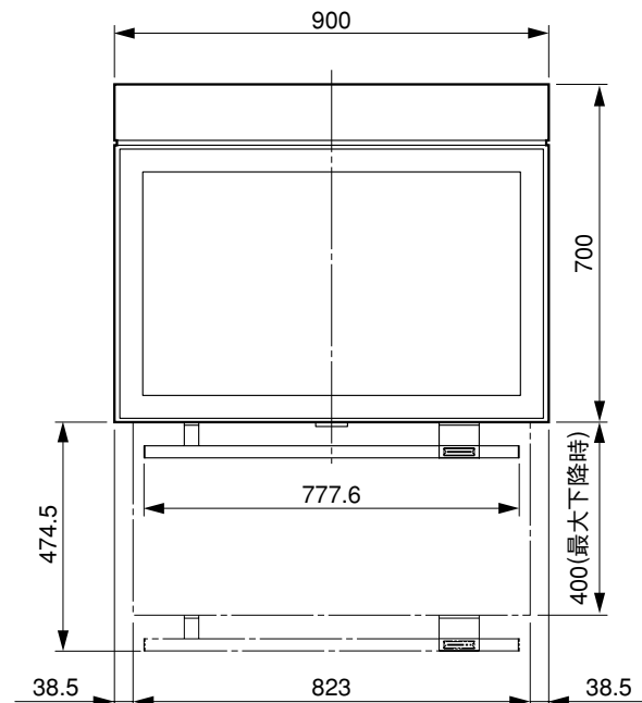
正面図
